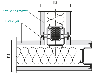
Т-образное примыкание под углом 90°
